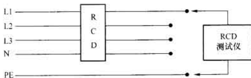
图 1 测试方法
