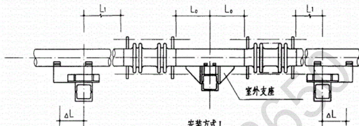
中间固定支架布置方式
