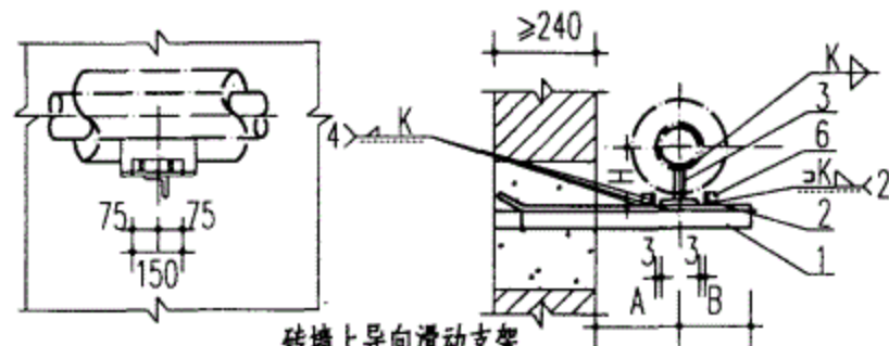
砖墙上导向滑动支架
