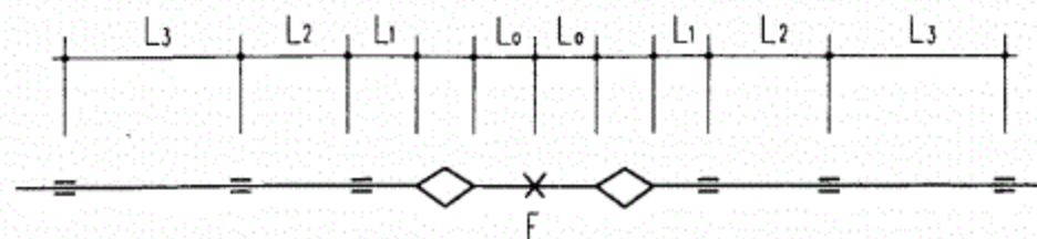
中间固定支架布置方式
