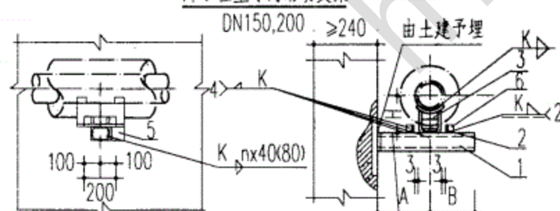
焊于柱上导向滑动支架
