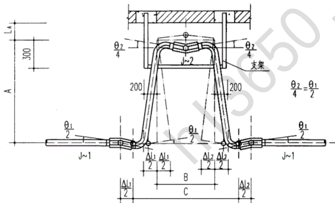
铰链型三铰点方型补偿单元安装详图(一)
