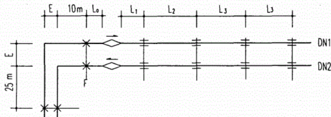
端部固定支架布置方式
