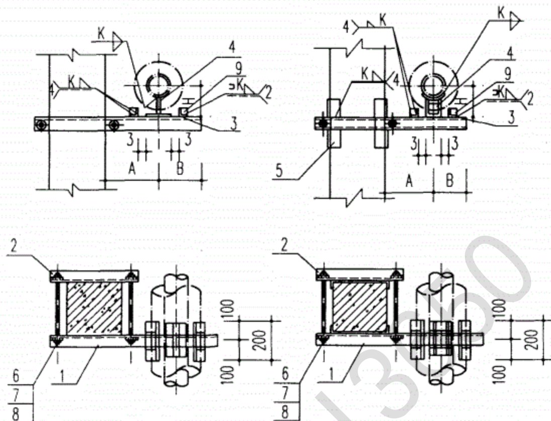
夹于柱上滑动支架 DN25~100
