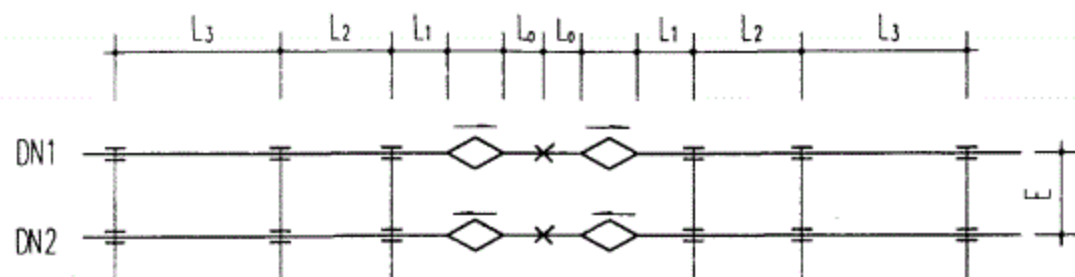
中间固定支架布置方式
