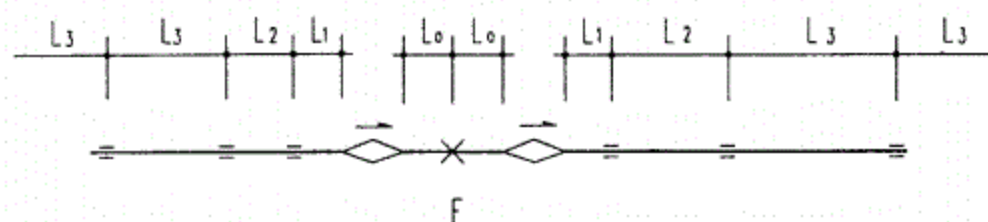
端部固定支架布置方式
